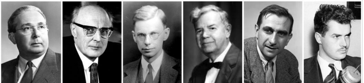
Leo Szilard
